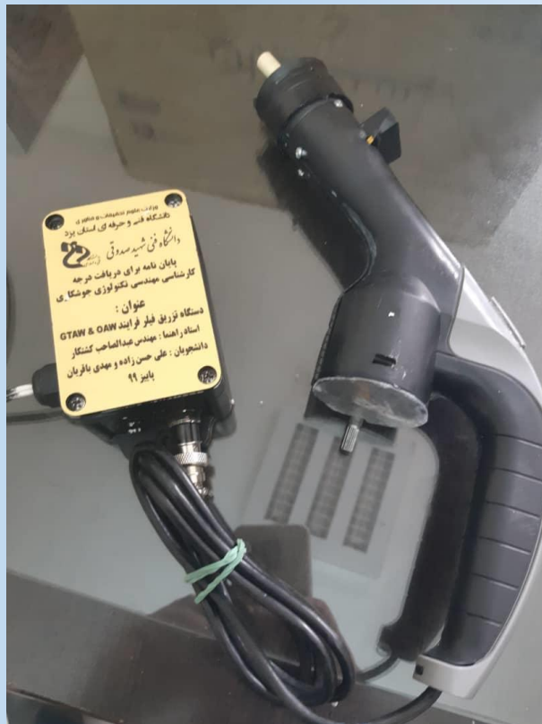
دستگاه تزریق فیلر فرایند OAW- CTAW
